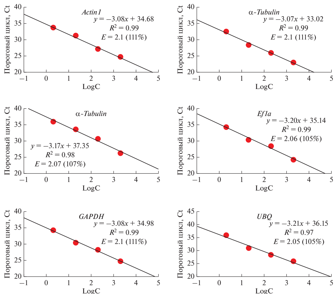
Рис. 2. Зависимость порогового цикла (Ct), полученного в ходе ПЦР для каждого референсного гена, от логарифма концентрации ДНК матрицы (LogC). Точками обозначены средние значения пороговых циклов по трем повторам. На графике показано уравнение зависимости, коэффициент корреляции ( R^2 ) и эффективность реакции ПЦР ( E ).
